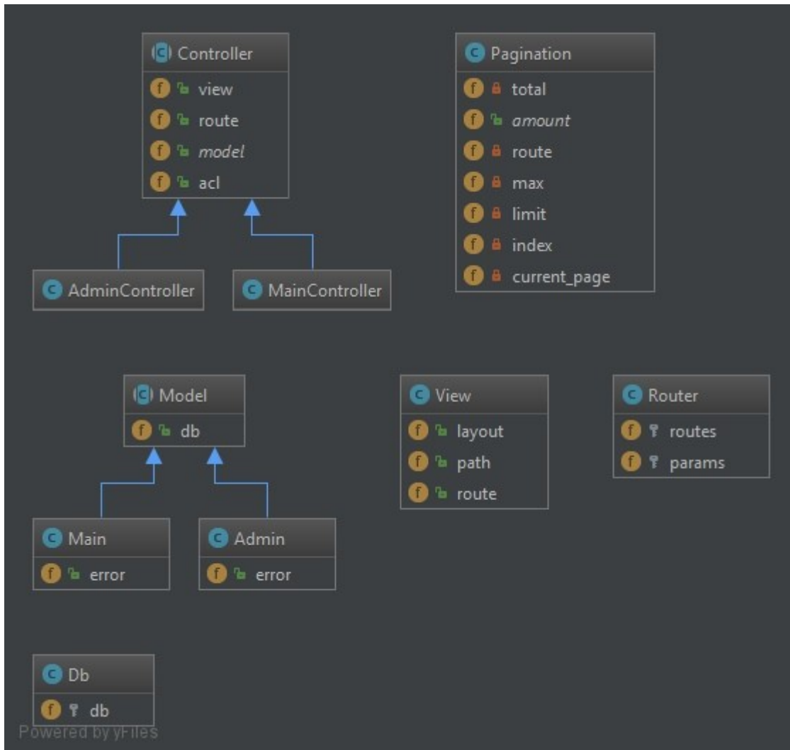
Рисунок 7.1 – Диаграмма классов
