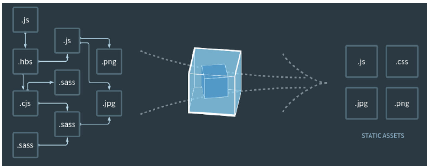
Рисунок 17 – Сборка Webpack
