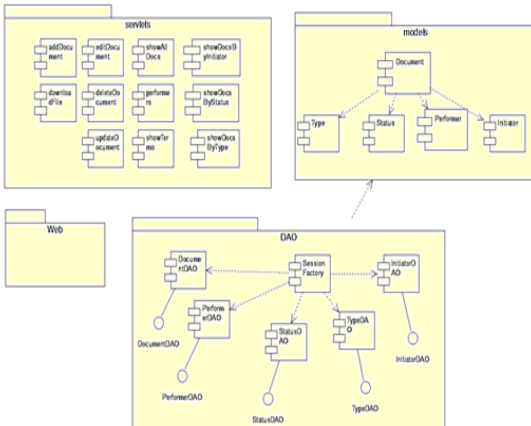
Рисунок 4.1 - Интерфейс Unity
